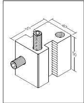
Klemmstück
