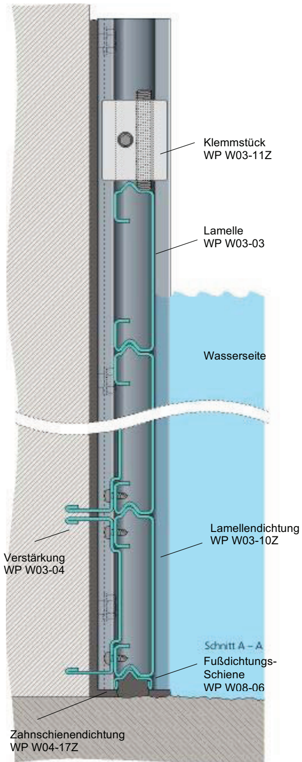
Seitenschnitt
